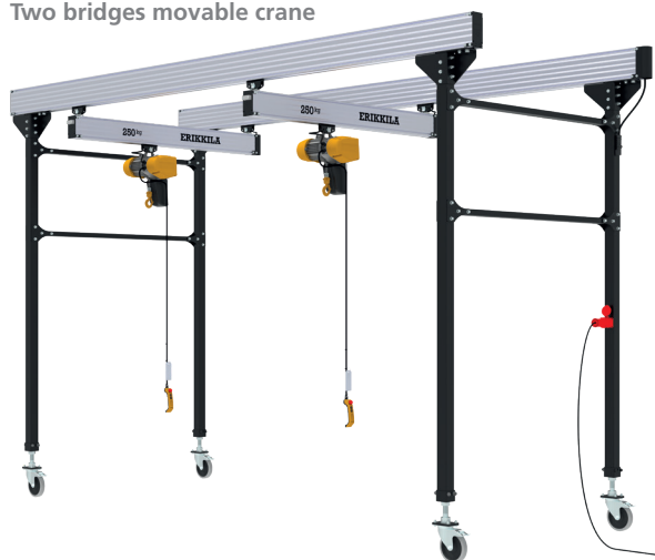
Gru mobile con due ponti Two bridges movable crane
