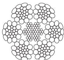
6x26KKWS+IWRC 205 fili/wires
